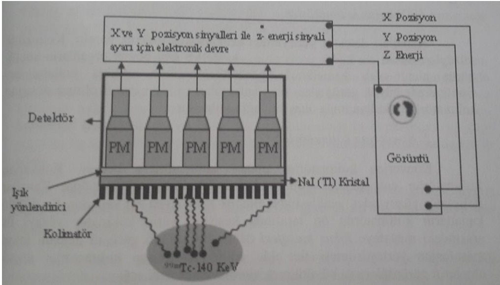
Şekil 2.3. Gama Kameranın İşleyiş Prensibi (Demir, 2008).
