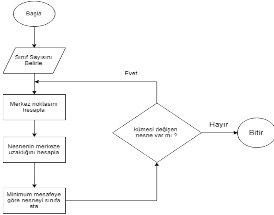
Şekil 2.2. K-means algoritması akış diyagramı
