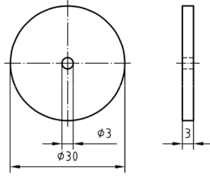
Şekil 3.21. DIN 13990-1/-2 standart formuna göre silikon kalıbın şematik görünümü (Şema formdan alınmıştır).
