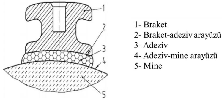
Şekil 3.4. DIN 13990-1/-2 standart formuna göre bağlanma dayanımının incelendiği elemanların kesitsel görünümü (Şema formdan alınmıştır).
