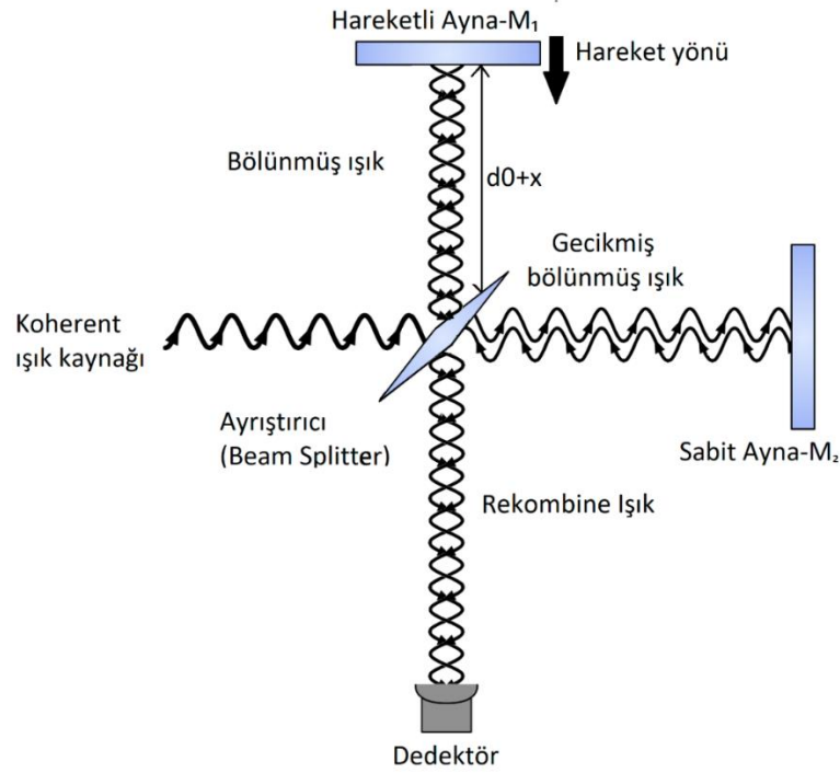
Şekil 2.32. Referans aynanın d_0+x uzaklığında olduğu durumda interferometrede ayrılan iki ışığın dedektöre yansımaları. M_1 ve M_2 aynalarından yansıyan ışınlar zıt fazlı koherent ve monokromatik olduğundan dalgalar birbirlerini sönmeler ve yıkıcı girişim oluşur.
