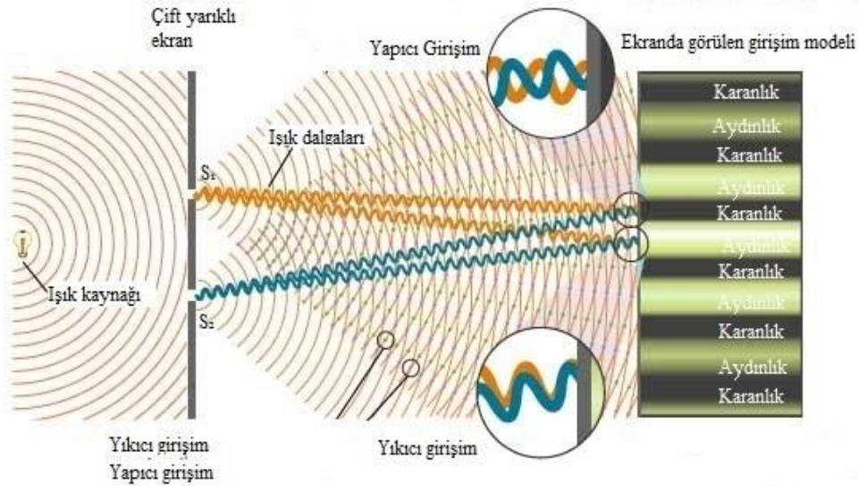
Şekil 2.29. Young deneyi, ışıkta girişim (116) .
