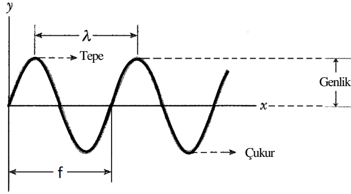
Şekil 2.26. Vektörel bir dalga. Dalgalar vektörel büyüklüklerdir. Tepe noktası y ekseninde dalganın en yüksek noktası, çukur noktası ise y eksenindeki en düşük noktasıdır. Bir tepe ile komşu tepe arasındaki uzaklığa \lambda dalga boyu denir. Birim zamanda verilen bir noktadan geçen tepelerin ya da çukurların veya dalga üzerindeki herhangi bir noktanın sayısıdır. Genlik ise bir ortamın bir parçacığının maksimum yer değiştirmesine denir (107) .
