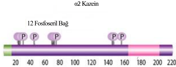
Şekil 2.16. Bir \alpha_2 kazein molekülü. Molekül üzerinde bulunan fosfoseril bağlar kalsiyum ve fosfat iyonlarını bağlar. (73)
