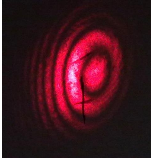
Şekil 2.31. Ekranaya yansıyan girişim deseni. Bu desende üst üste binen ışık dalgaları aydınlık, birbirini sönmüleyen ışık dalgaları karanlık alanlar olarak görünür (117) .
