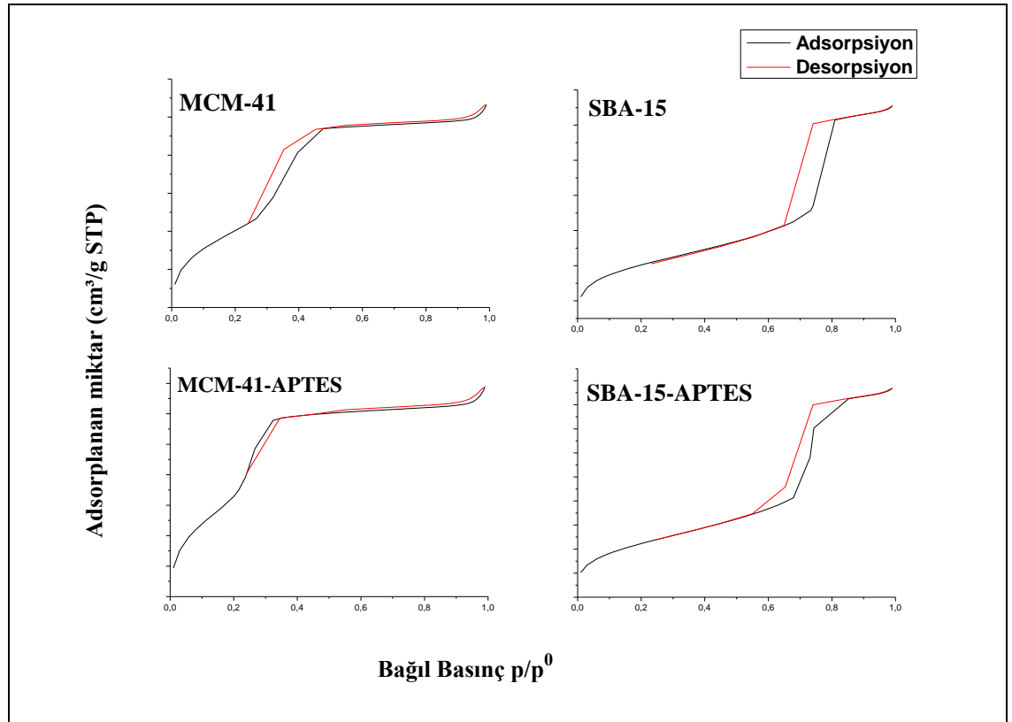
Şekil 4.14. Yalın ve APTES modifiye MSN'lere ait N 2 adsorpsiyon-desorpsiyon izotermleri
