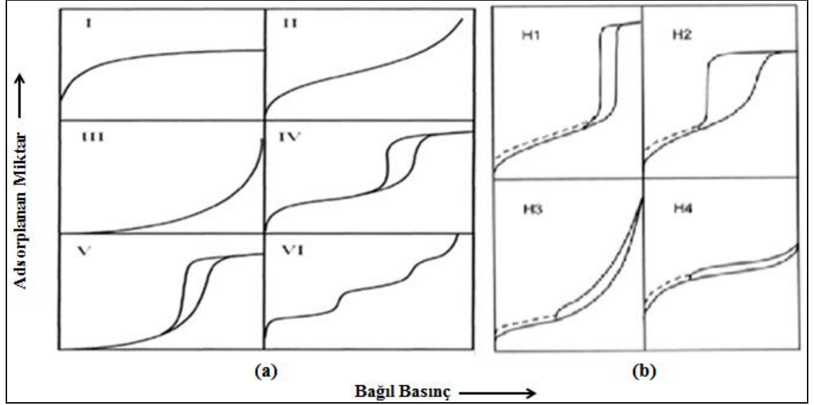
Şekil 4.13. (a) Adsorpsiyon-desorpsiyon izotermlerinin IUPAC sınıflandırması ve (b) izotermlerin gözenek şekli ile ilişkisi
