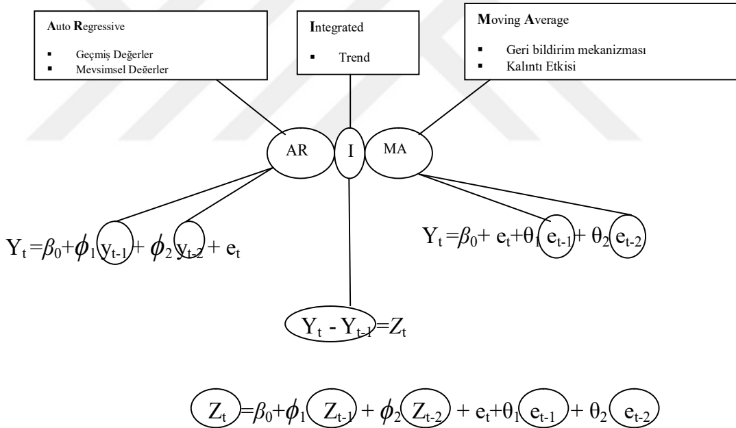
Şekil 1.2 Otoresif Bütünleşik Hareketli Ortalama (ARIMA) Modeli
