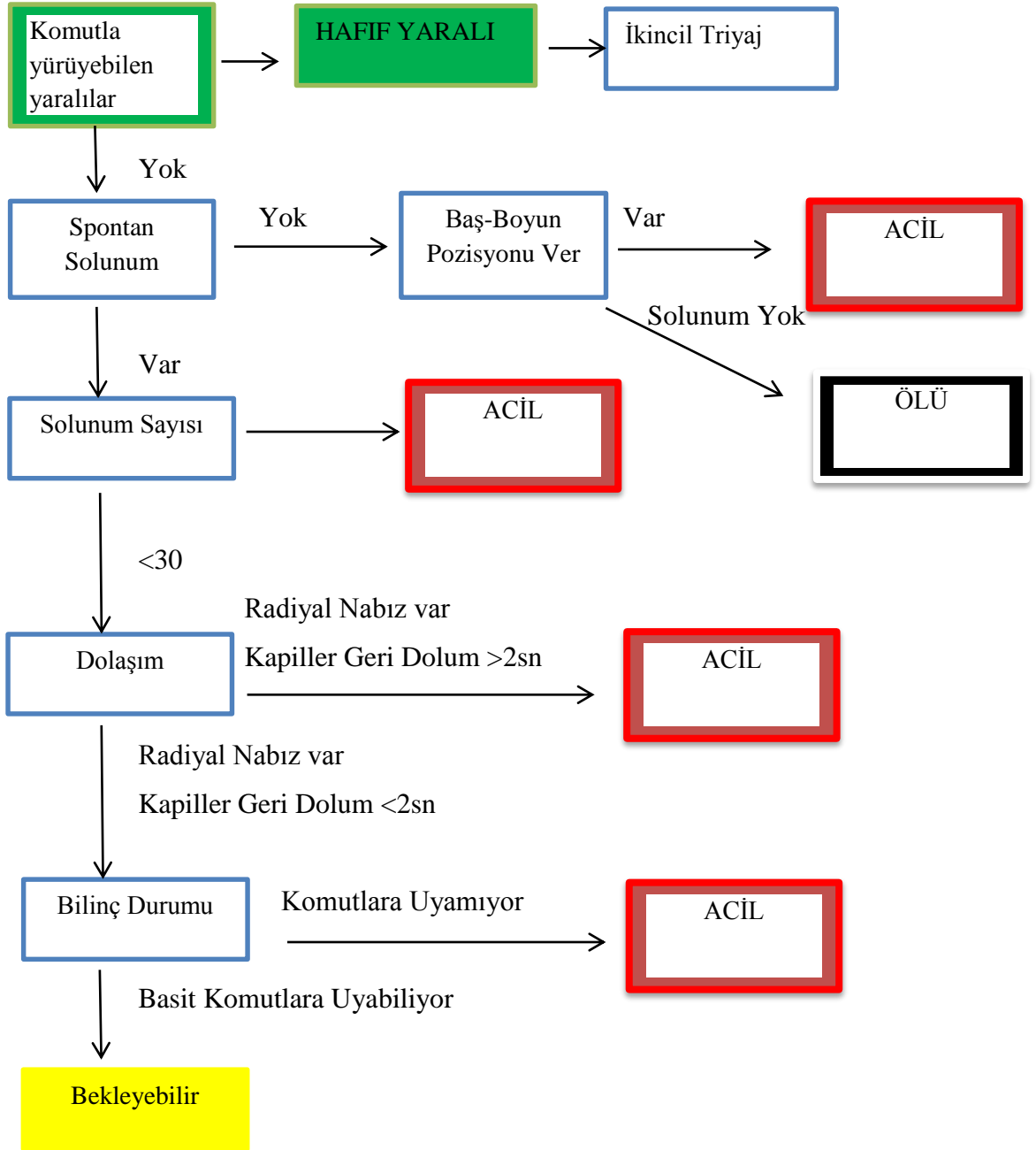
Şekil 2.1. START Algoritması
