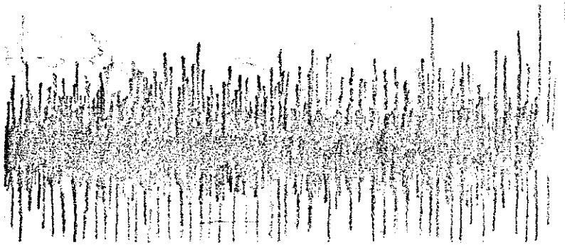
İnterferans örneği
