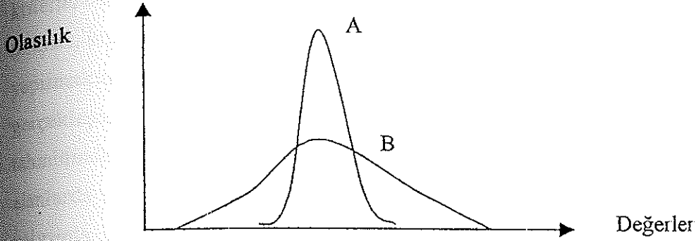
Şekil 2.9 Dağılımların basıklığı
