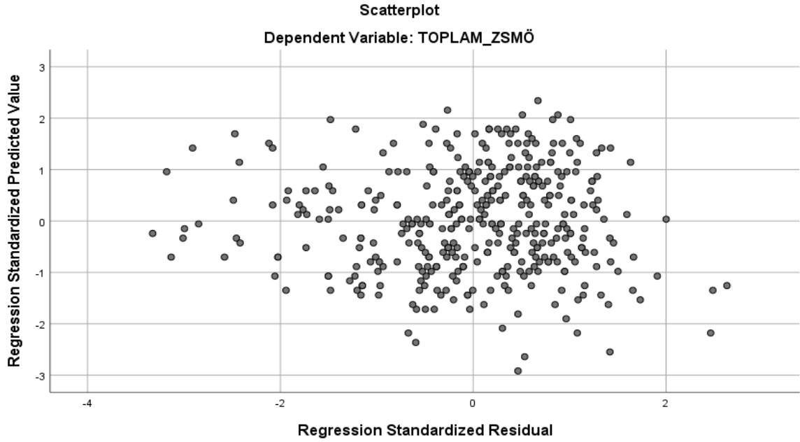
Şekil 3.3. Regresyon Modeli için Artıkların (Rezidüellerin) Saçınıtı Grafiği (Bağımlı Değişken = Zorbalığa Seyirci Müdahalesi Puanları)
