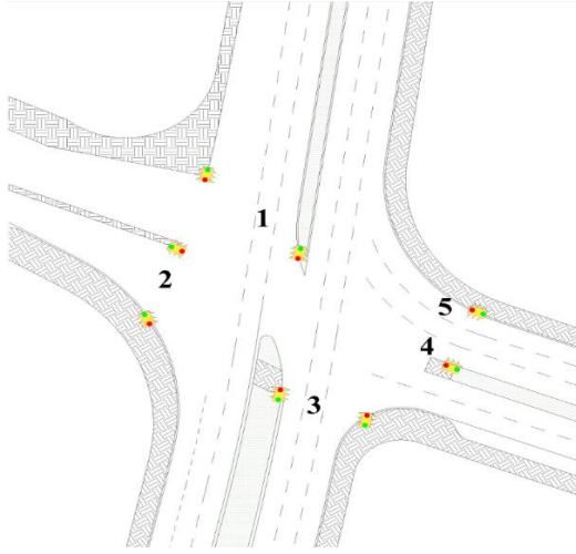
Şekil 4.4. Balıkçioğlu-Narenciye Kavşağı trafik ışıkları planı (2016)
