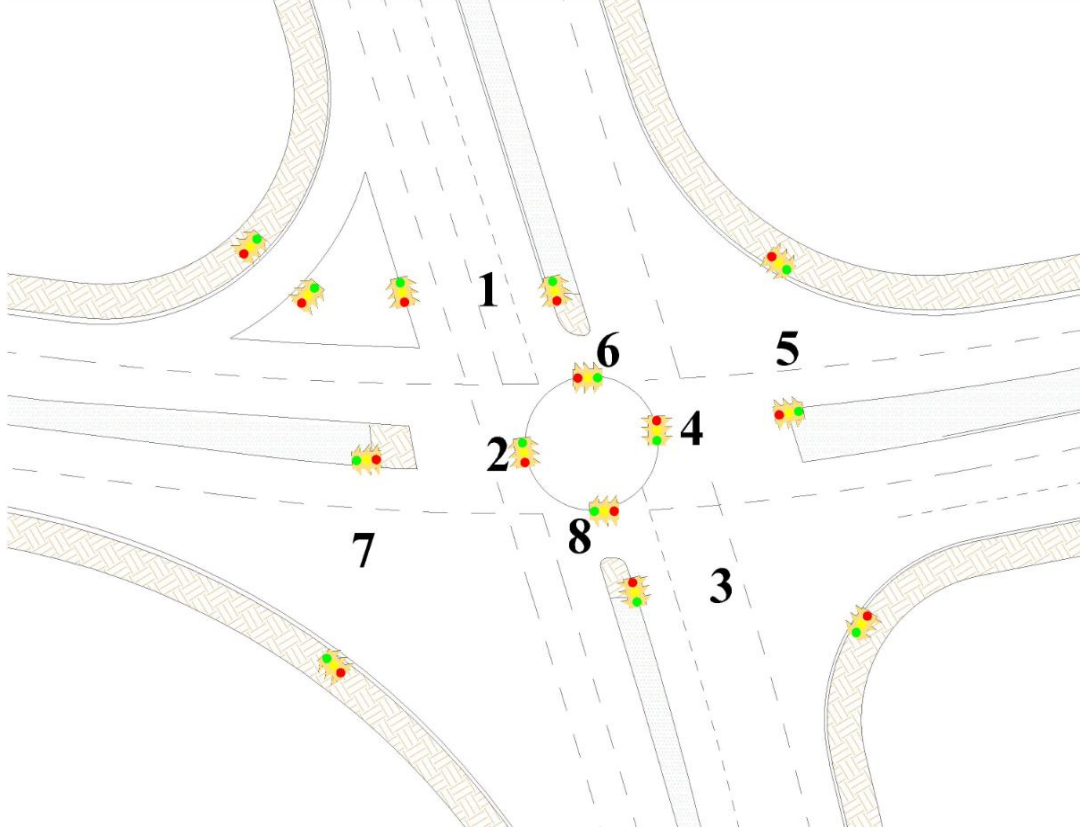
Şekil 4.6. Sampi Kavşağı trafik ışıkları planı (2016)
