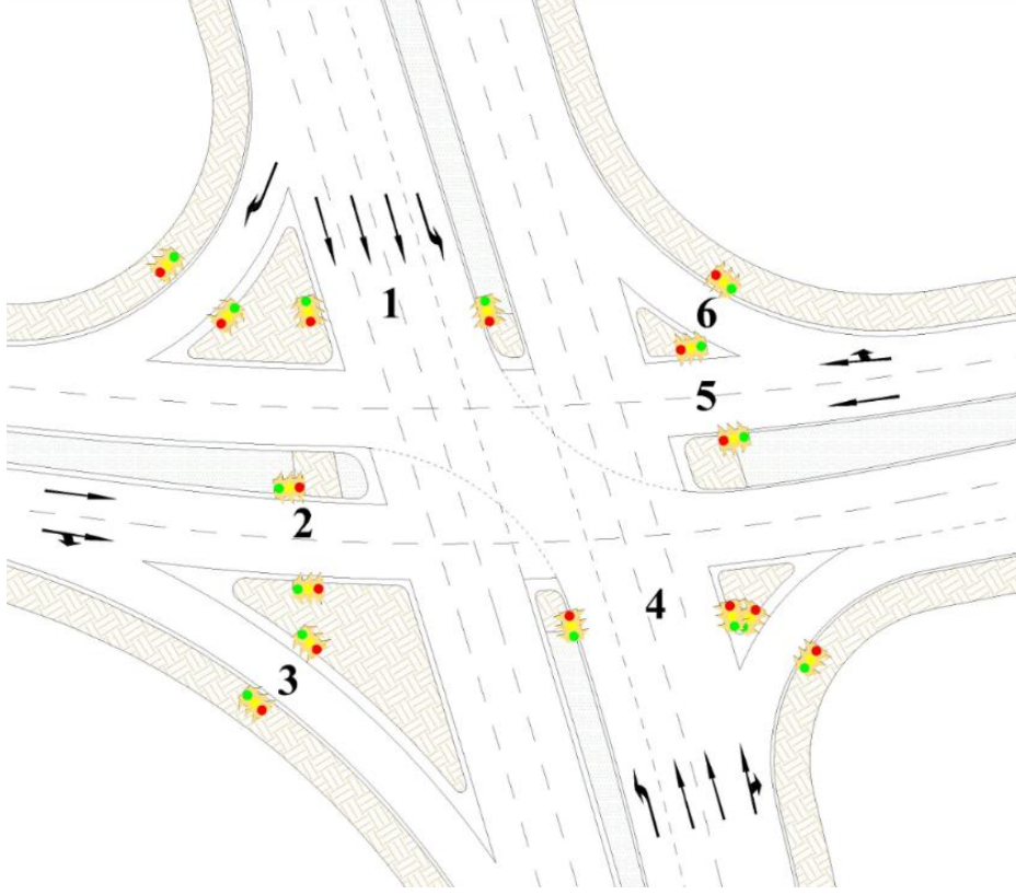
Şekil 4.23. Sampi Kavşağı trafik ışıkları planı
