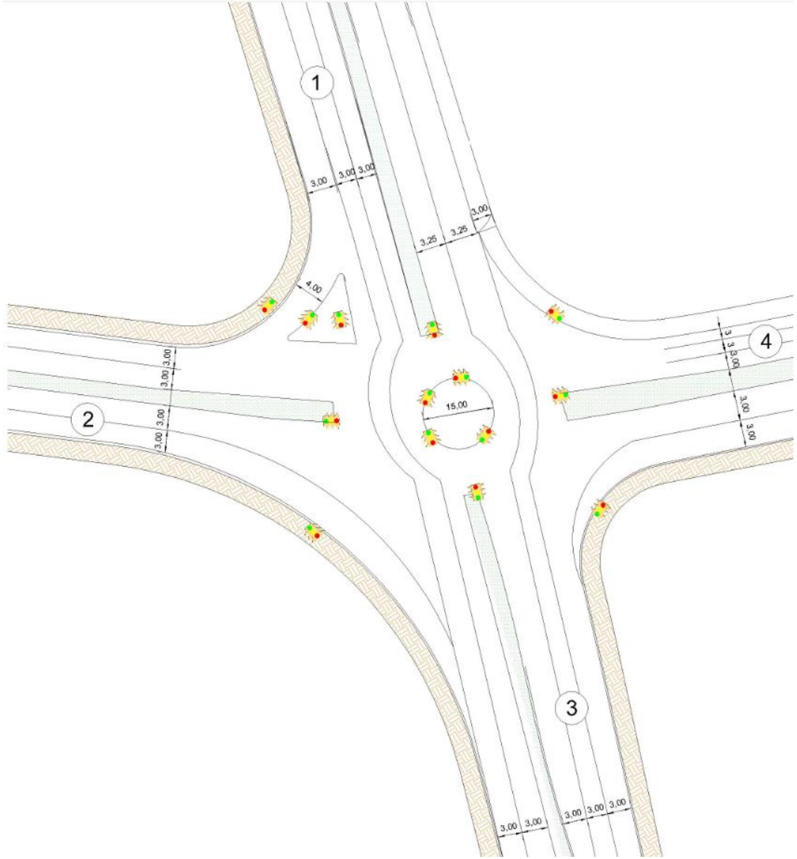
Şekil 3.5. Sampi Kavşağı rölöve planı (2016)
