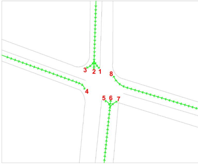
Şekil 4.8. Balıkçioğlu - Narenciye Kavşağı araç sayım planı
