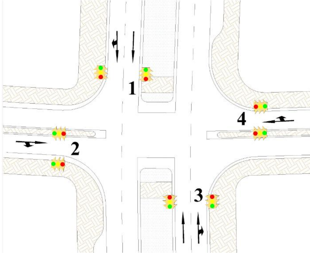
Şekil 4.21. Komaş Kavşağı trafik ışıkları planı
