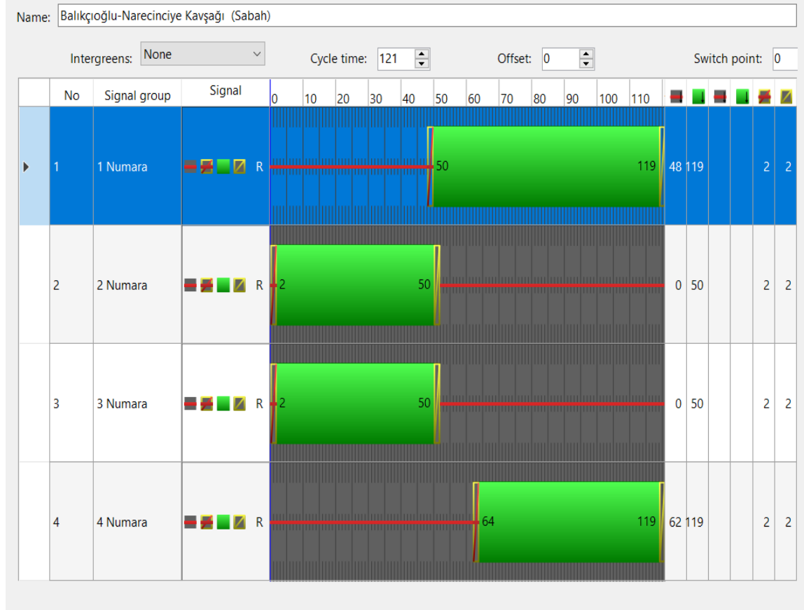
Şekil 4.19. Balıkçıoğlu-Narenciye Kavşağı 20.00 – 16.00 arası sinyal zaman diyagramı
