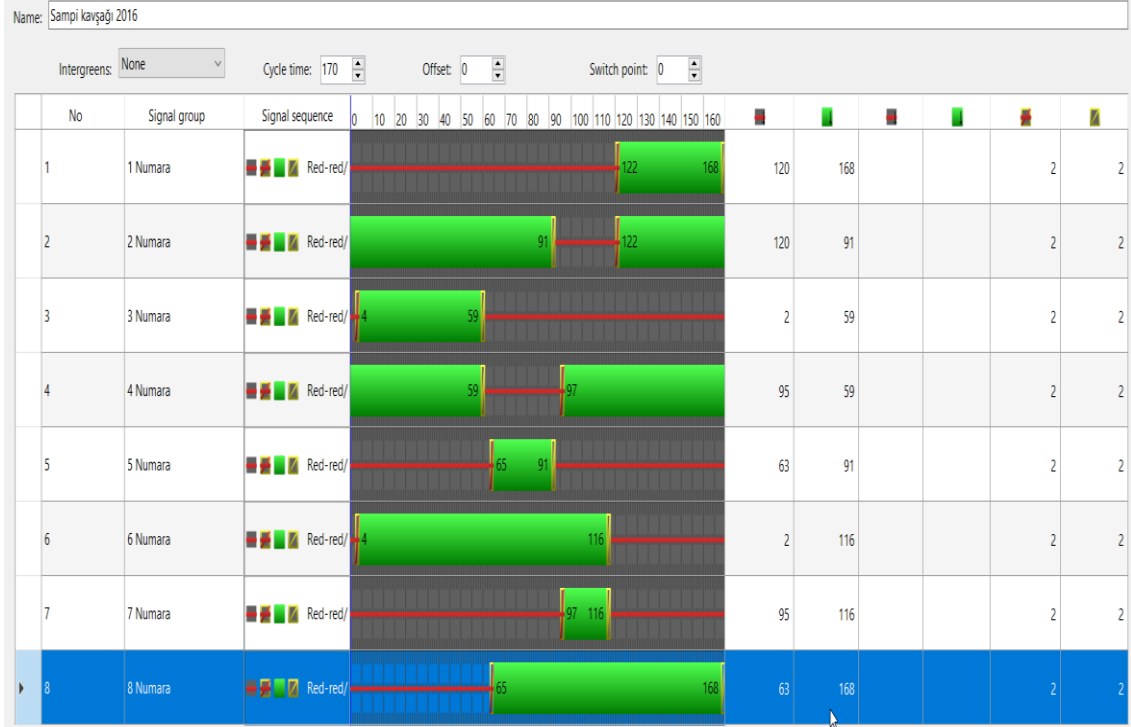
Şekil 4.7. Sampı Kavşağı sinyal zaman diyagramı (2016)
