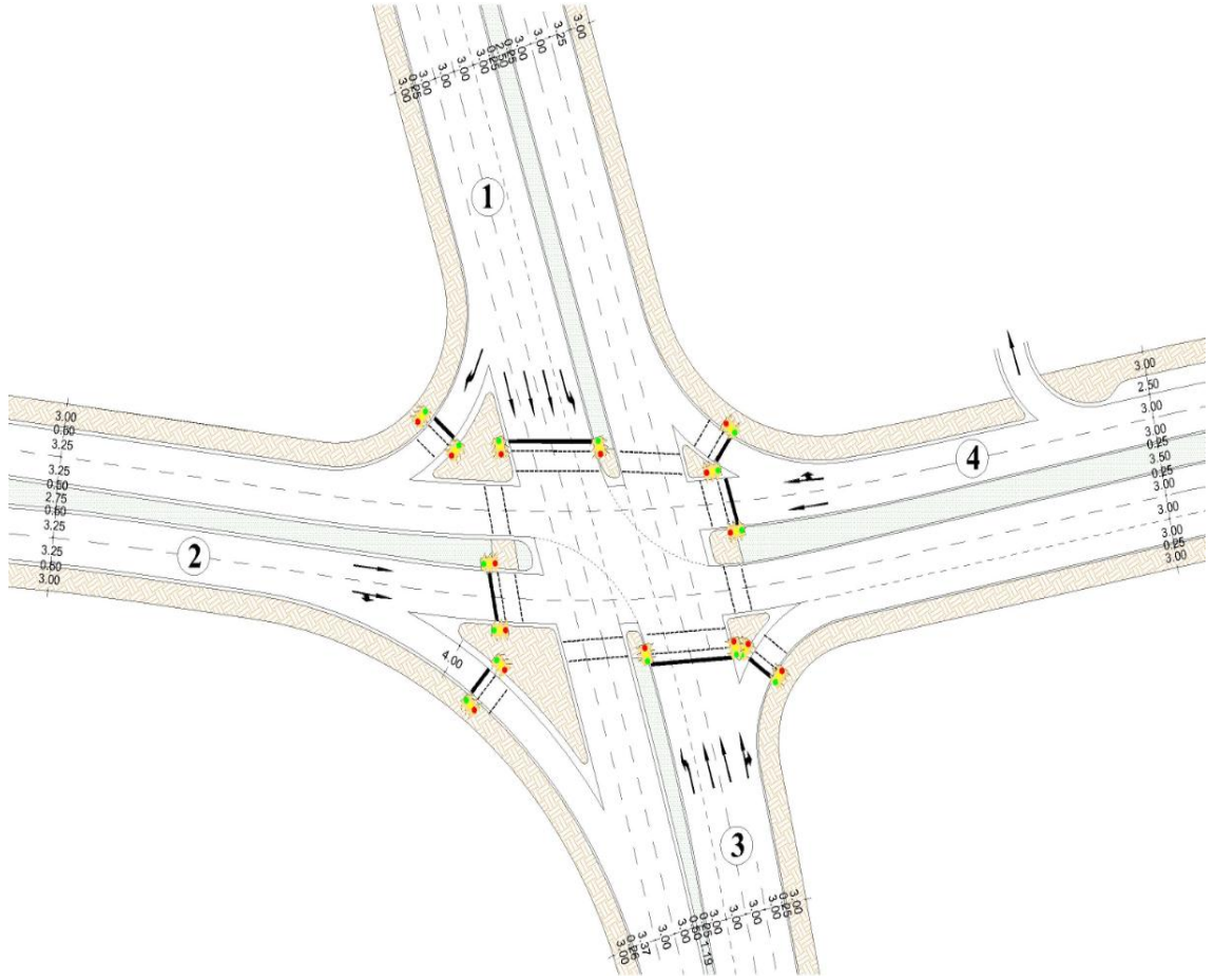
Şekil 3.15. Sampi Kavşağı rölöve planı
