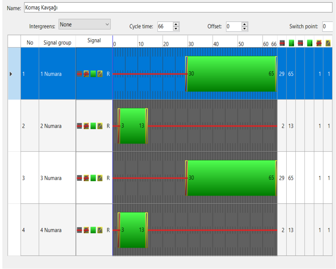
Şekil 4.22. Komaş Kavşağı sinyal zaman diyagramı
