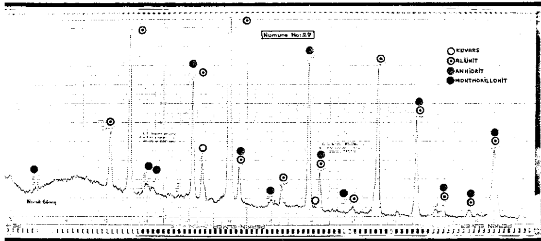
Şekil 27. Değirmendere'den alınan 27 No'lu örneğin X-ışınları kırınım grafiği
