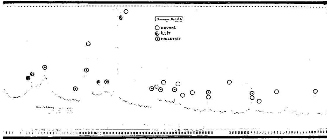
Şekil 26. Değirmendere'den alınan 26 No'lu örneğin X-ışınları kırınım grafiği
