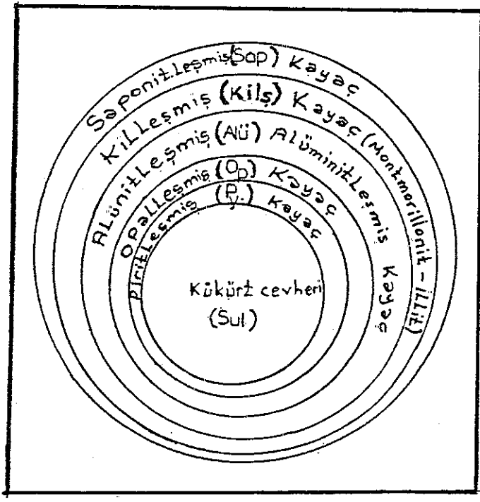
Şekil 18. Mineralleşme merkezinin veya cevher kütlesinin etrafındaki altere kayaların zonal düzenlenmesini gösteren idealleştirilmiş şema Mukaiyama (1988)'den esinti.
