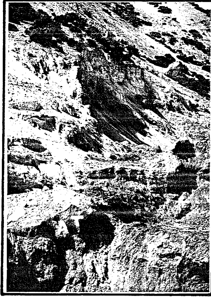
Şekil 9. Kokardere kesiminde yüzeylemiş andezitik tüfler (AT).
