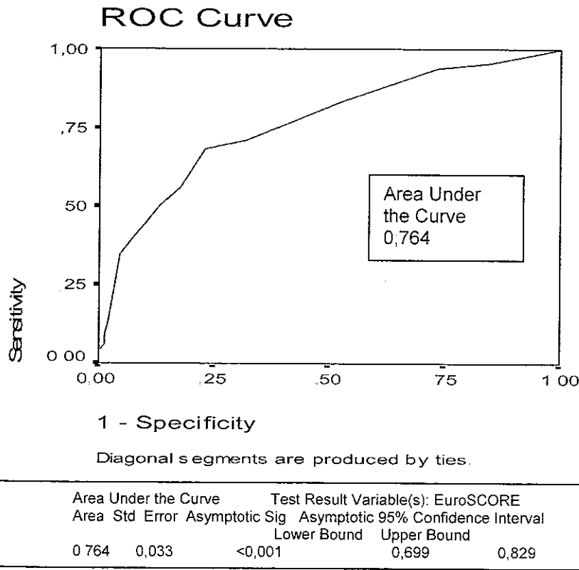
Şekil – 5.2: EuroSCORE risk sistemi ile hastalarımızın ROC eğri analizi
