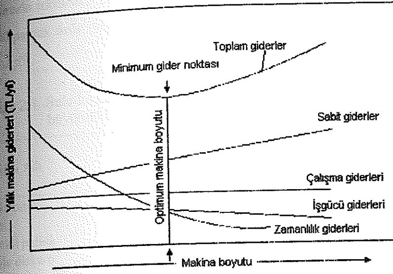
Şekil 2.5. Makina giderlerinin makina büyüklüğü ile değişimi (Işık 1988)
