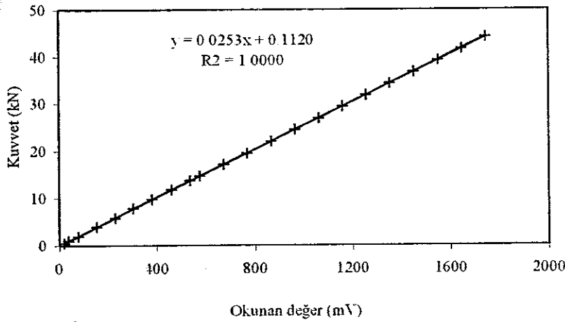
Şekil 3.6. Çeki dinamometresi kalibrasyon grafiği ve regresyon eşitliği
